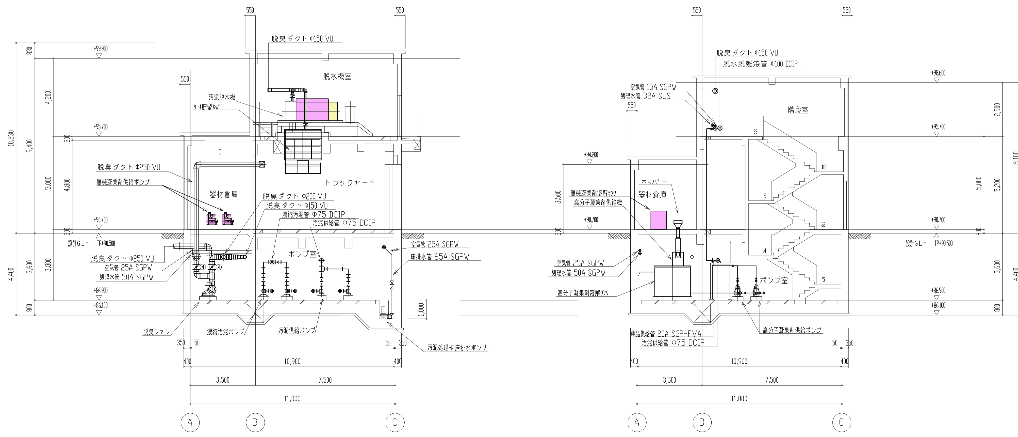
C-C 地断面図 1/100
