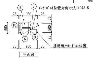
1階 平面図 S=1/100
