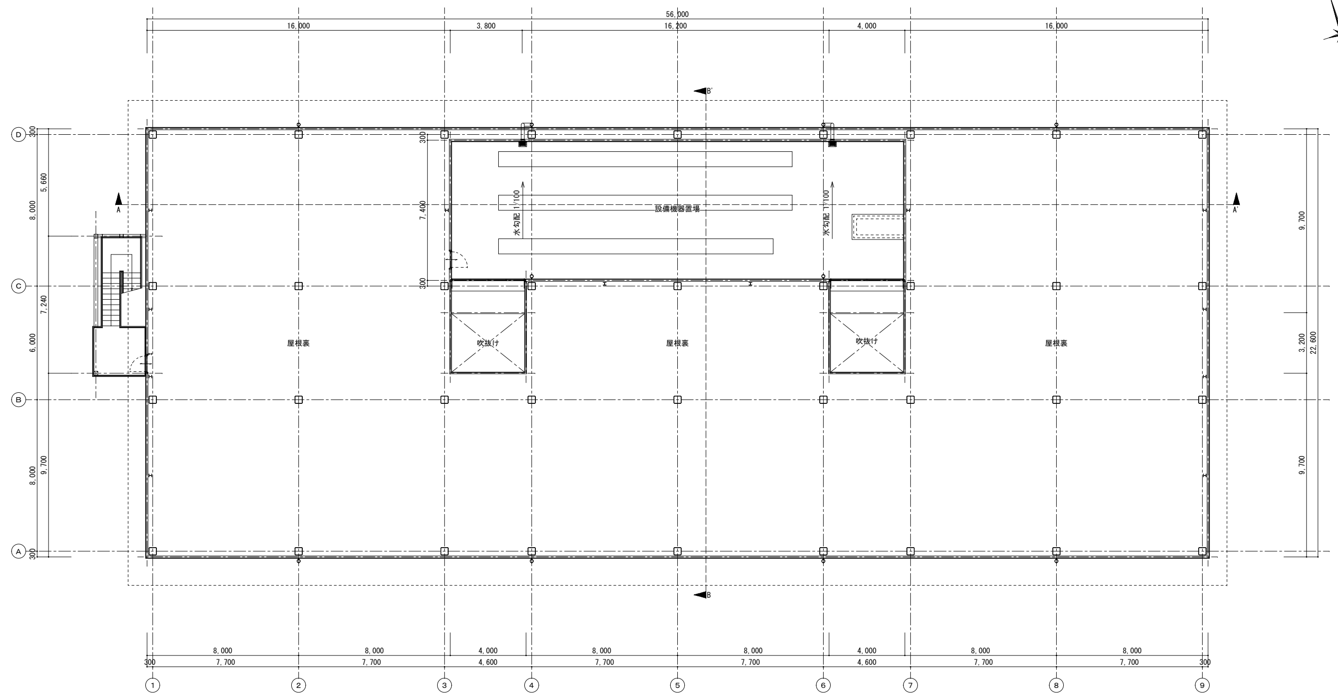
R階 平面図 S=1/100
