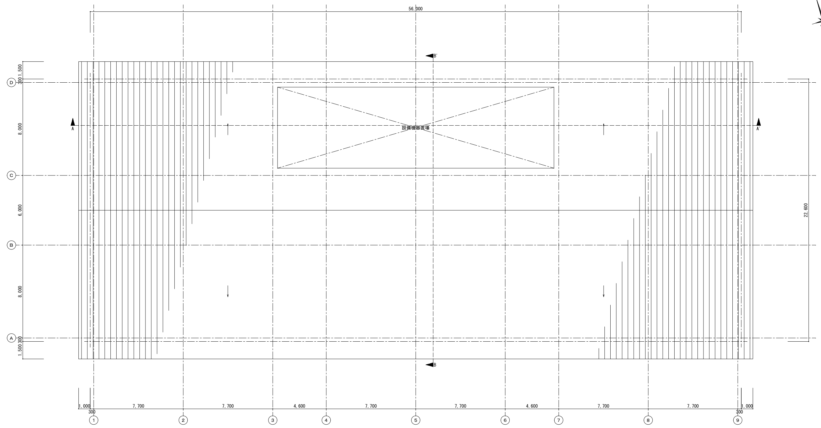
屋根伏図 S=1/100
